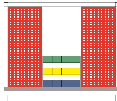
RH & LH (min table width >1400 mm)
